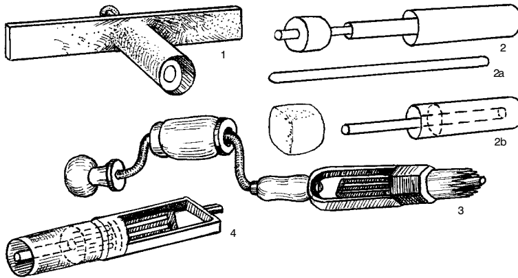
10 pav. Prietaisai plūdėms daryti: 1 – plūdei iš putplasčio išpjauti. Jurbarko r., Viešvilės k.; 2 – skylėi plūdėje išpjauti (b), išpjautam gabaliukui išstumti (a). Jurbarko r., Viešvilės k.; 3 – ranka sukamas prietaisas. Šakių r., Kidulių k.; 4 – elektra sukamas prietaisas. Jurbarko r., Molynės k.
