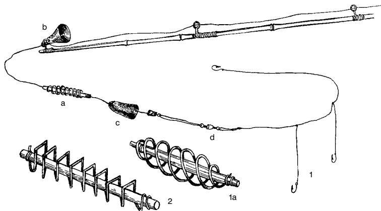
13 pav. Spiningas: 1 (a – šėrykla, b – skambutis, c – švinas, d – suktukas). Jurbarko r.; 2 – šėrykla. Šakių r.
