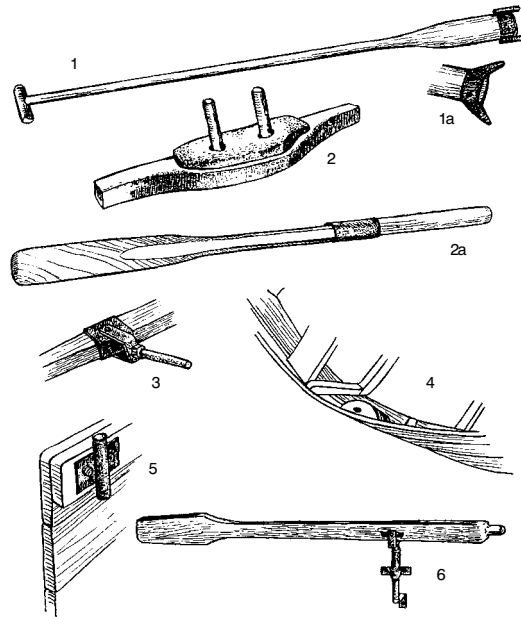
20 pav. Irklai: 1 – stumiamasis. Kauno r., Pelenių k. 1a – apkausto forma. Jurbarko r., Molynės k.; 2 – trinkelė su pirštais įdedamajam irklui (2a – įdedamasis irklas). Veliuona; 3 – irklo metalinis pirštas. Kelmės r.; 4 – medinė trinkelė vidinėje valtys pusėje. Trakų r.; 5 – metalinis vamzdelis irklui įstatyti. Zarasų r.; 6 – irklas vamzdelinėje apkaboje. Rokiškio r.
