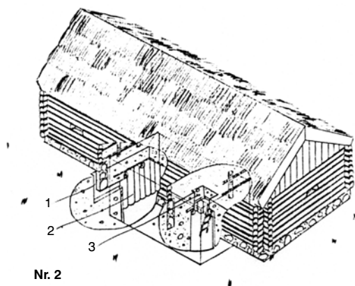
Pastatas Nr. 2: 1 – ventiliacinė anga; 2 – žeminė; 3 – landa į žeminę iš gardo
